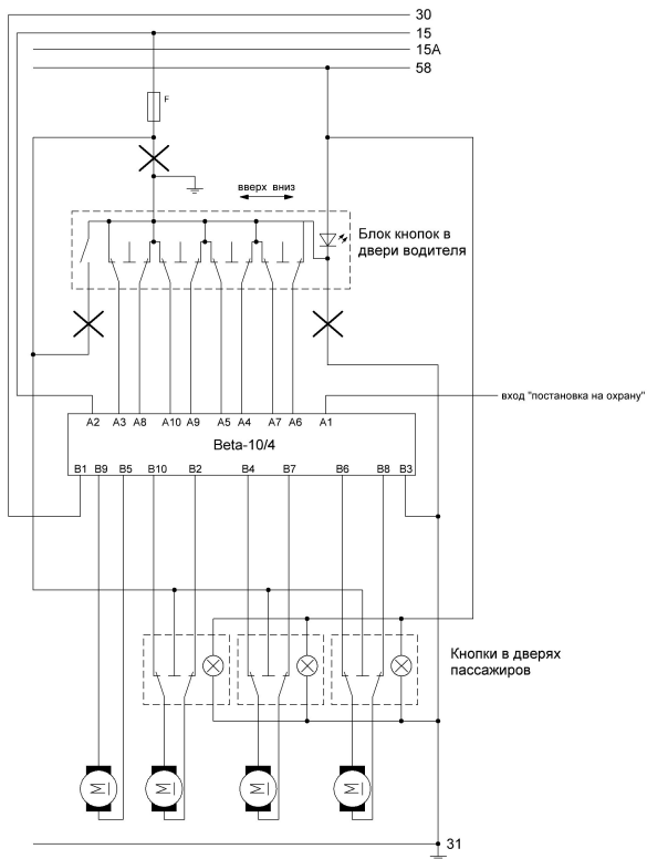
Схема подключения Beta-10 на Daewoo Nexia и др. а/м с аналогичной схемой подключения кнопок.
